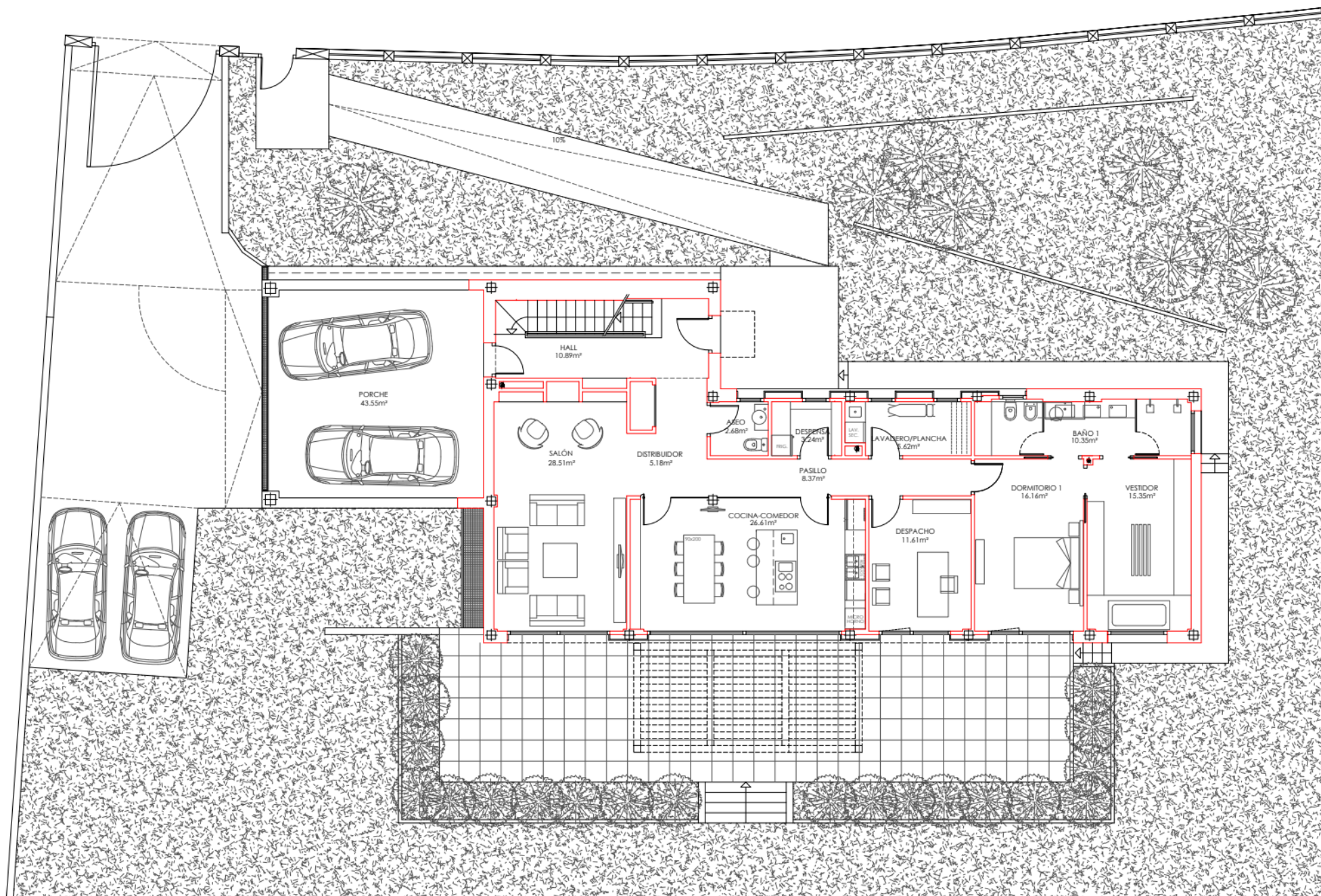
PLANTA BAJA
